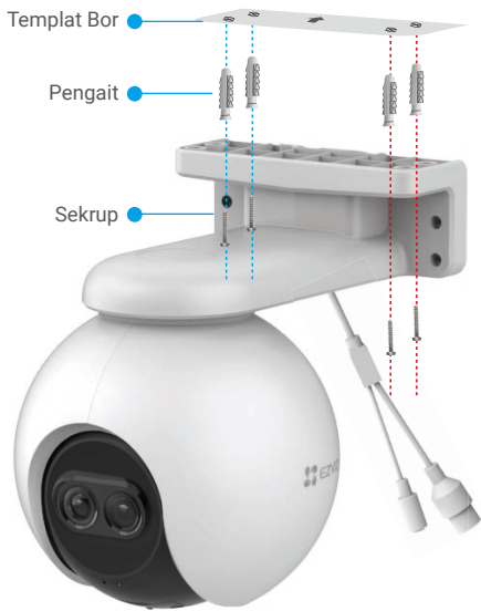
Gbr. 1 Pemasangan pada Plafon
