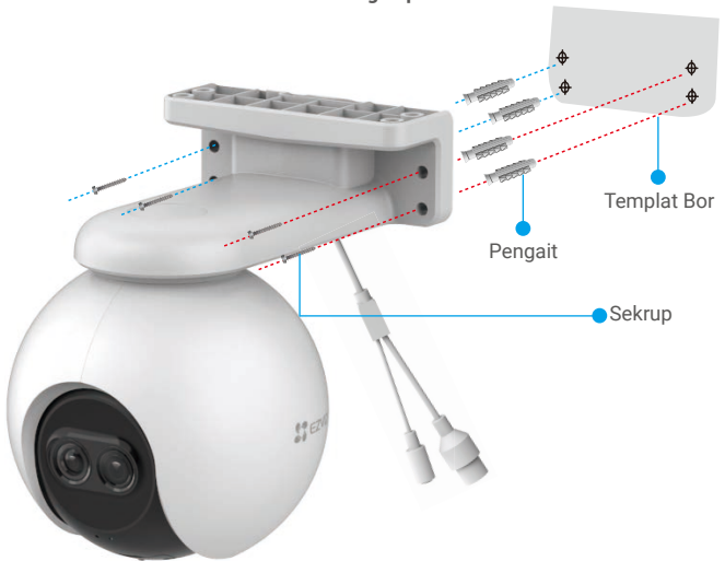
Gbr. 2 Pemasangan pada Dinding
